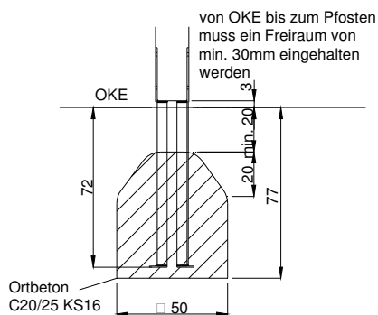
Fundamentschnitt Pfostenschuheinbau
