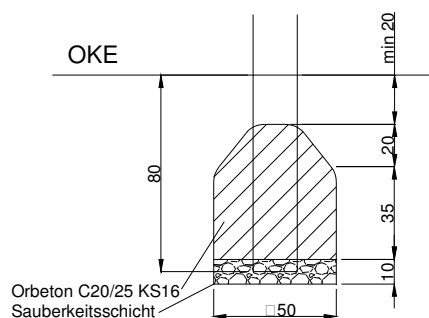
Fundamentschnitt Robinien-/ Douglasienpfosten
